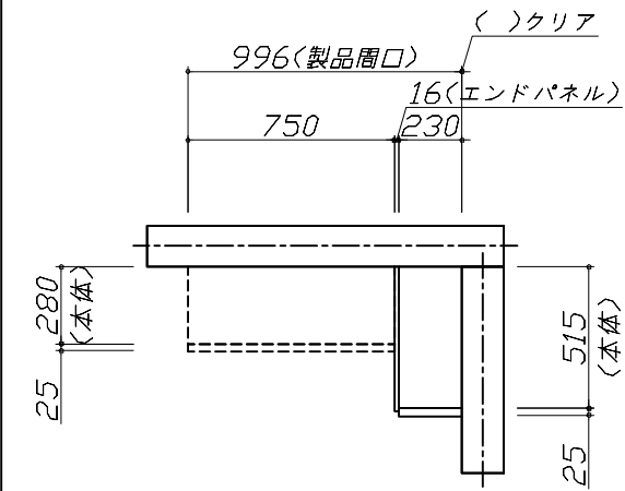
上台伏せ図
