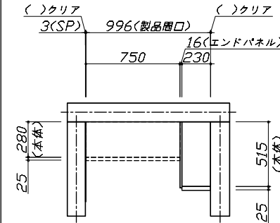
上台伏せ図
